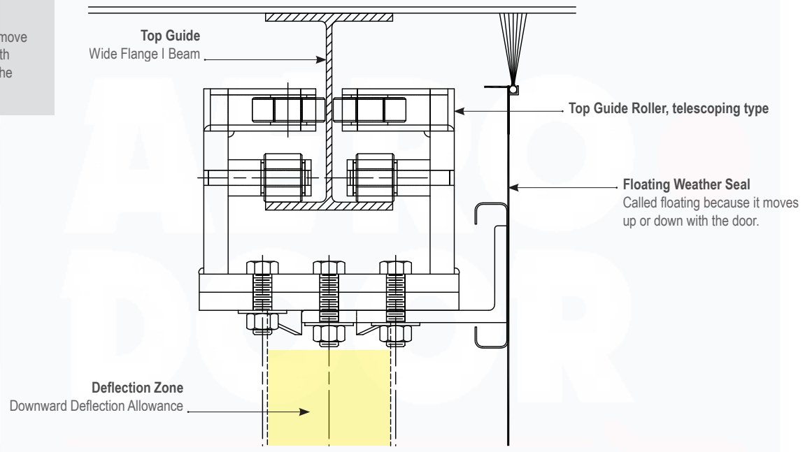
1 TOP GUIDE DETAIL SCALE: N.T.S.
