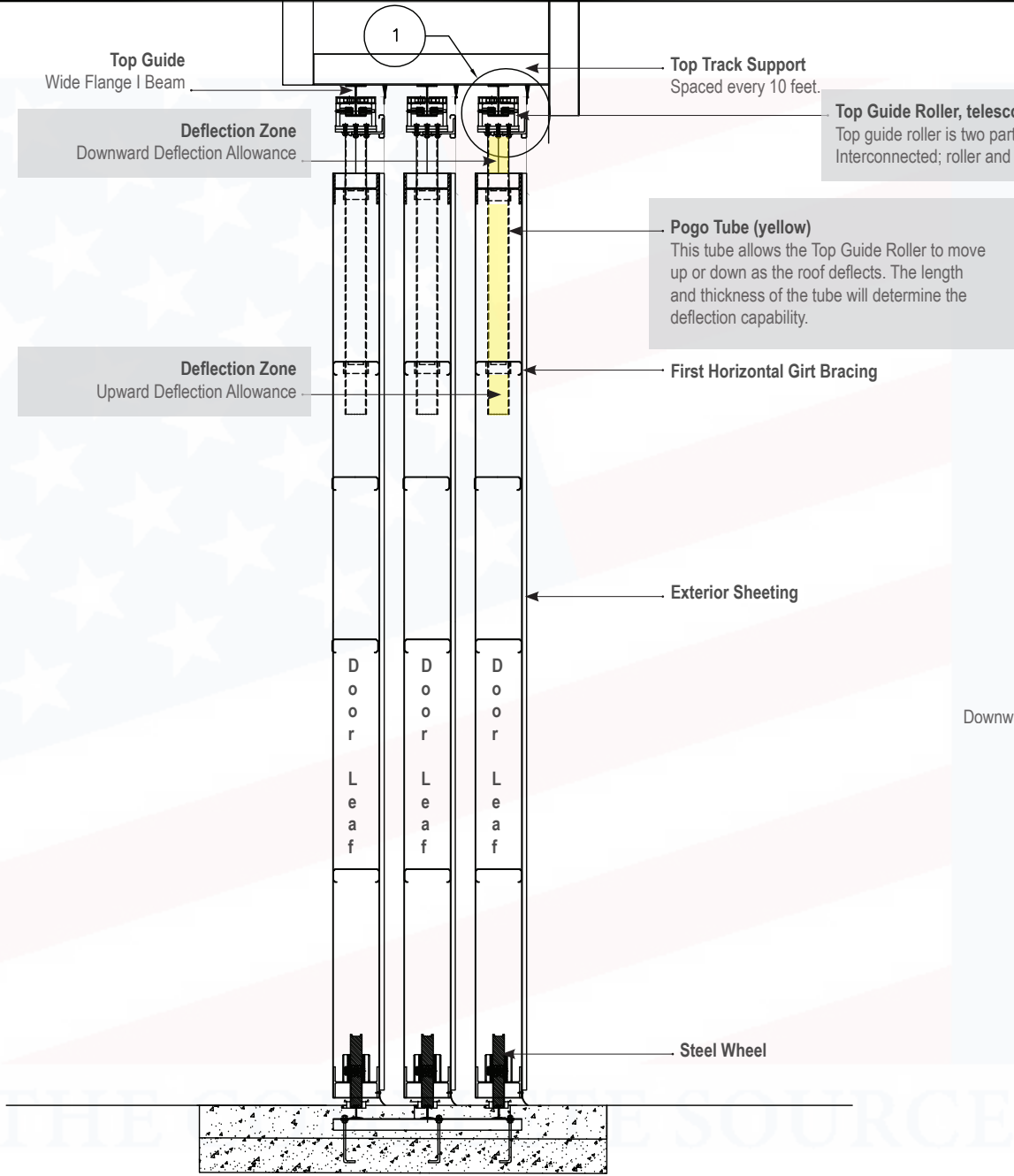
1 TOP GUIDE DETAIL SCALE: N.T.S.
